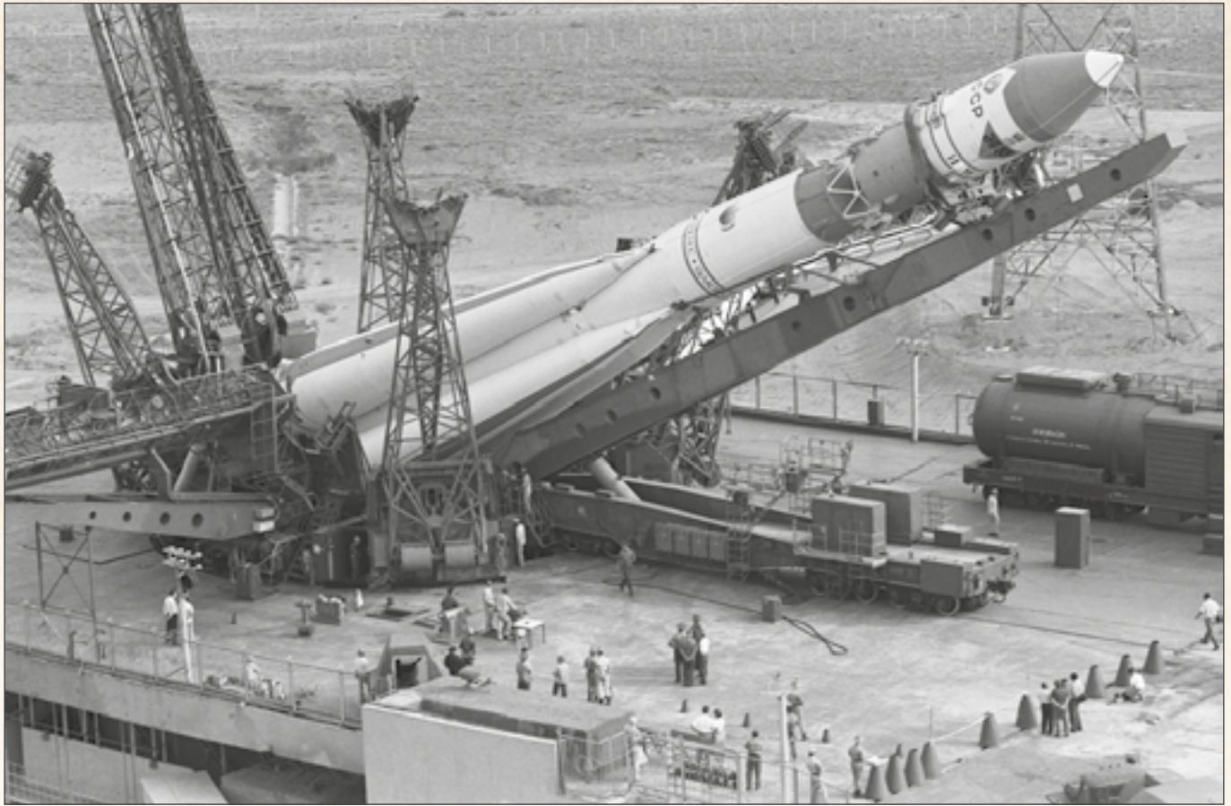
▲ Ракета Р-7
