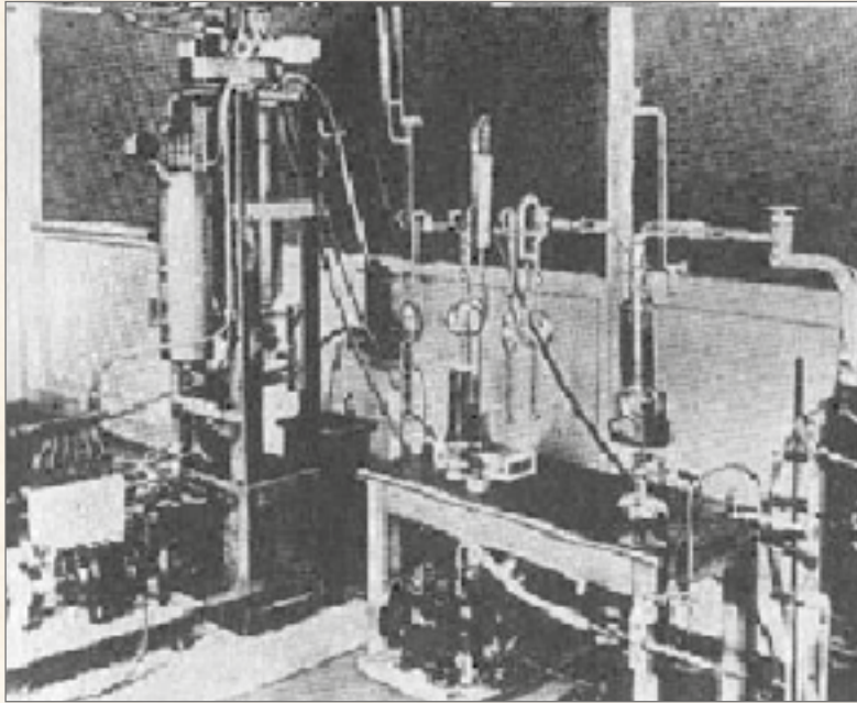
▲ Первая ультрацентрифуга, построенная Хартеком и Гротом для обогащения урана-235
