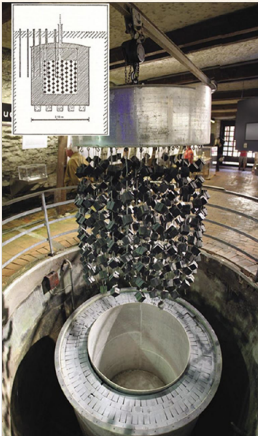
▲ Урановый реактор Рейха
